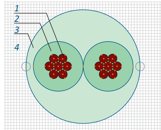
Рис. 5. Расчётная модель двухжильного кабеля для примера 2: 1 – 7-проволочные проводники; 2 – изоляция проводников; 3 – изолирующая оболочка; 4 – окружающая среда
