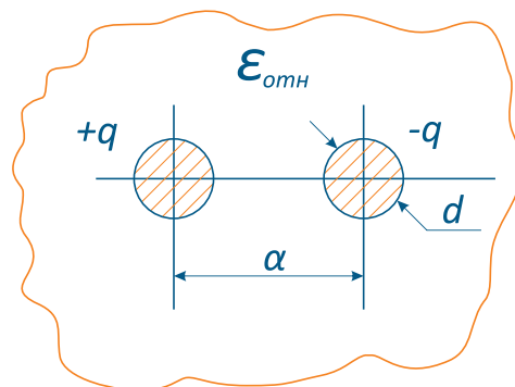
Рис. 1. Двухпроводная цепь с удалёнными проводниками
