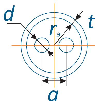
Рис. 7. Схема двухжильного экранированного кабеля
